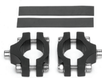
LM-1 Montageset für Gabeln ohne Ösen Art. 72100
